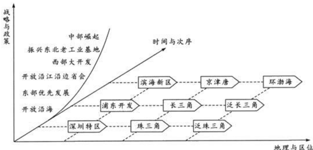
图3 改革开放以来中国区域发展的梯次开发模式
