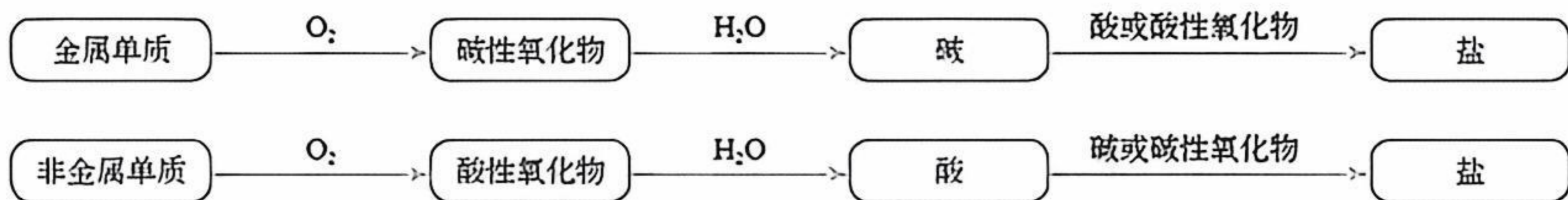
图：单质到盐的一种转化关系
