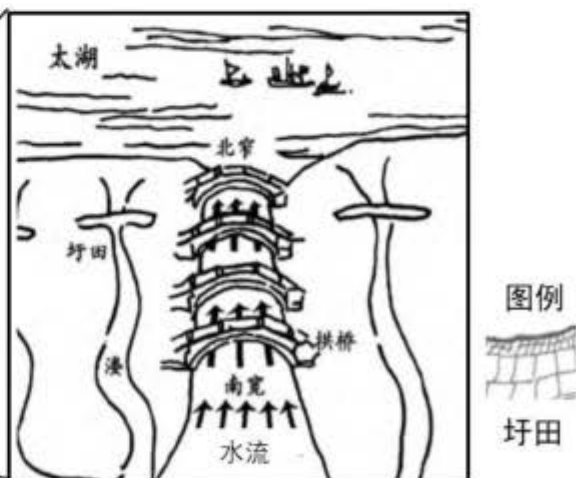
“束水攻沙”水利设施示意图
