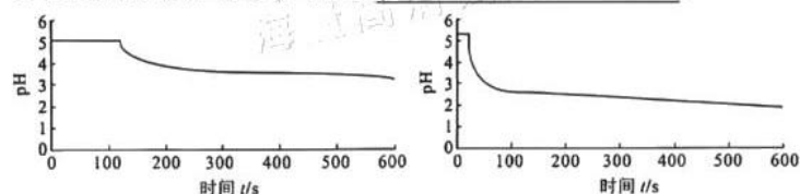
\text{SO}_2 通入 \text{Ba}(\text{NO}_3)_2 溶液(无氧)中的 pH-t 曲线
